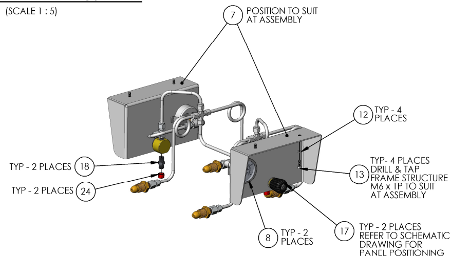
(SCALE 1 : 5)
