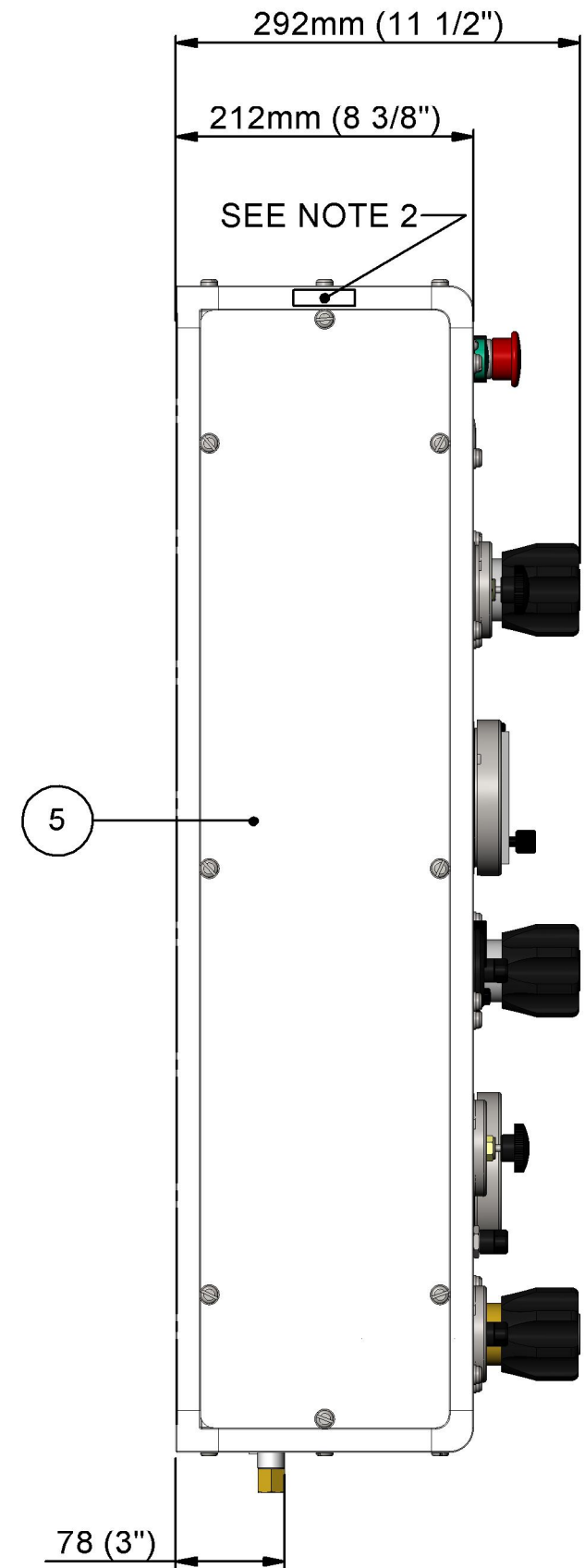
END ELEVATION
